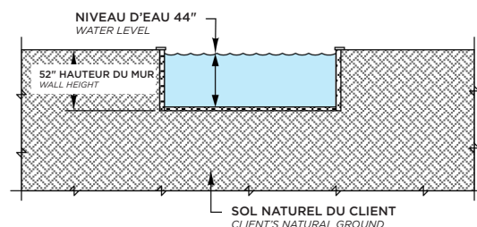
TRÉVI PRESTIGE installée sur un terrain plat TREVI PRESTIGE installed on a flat terrain
