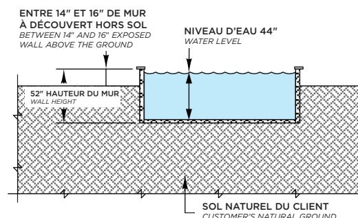
TRÉVI EUROPEA quatre côtés de mur exposés à 16" du sol
