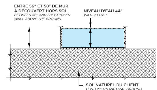
TRÉVI FUTURA quatre côtés de mur exposés à 56" du sol
