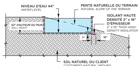
TRÉVI PRESTIGE EXPOSÉE un à trois côtés de mur exposés à plus de 24" du sol
